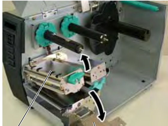
打印头模块
